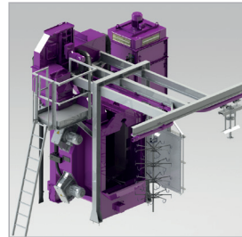
AGTOS hangbaan
